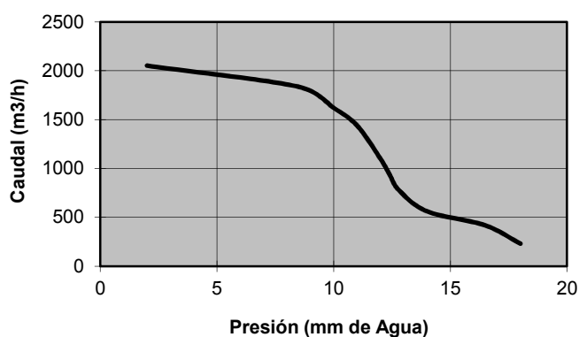
Curva Presión/Caudal
